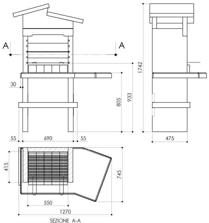
SEZIONE A-A
